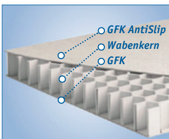
Schema 18 mm Wabenkernboden
