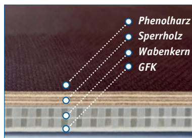
Boden 18 mm mit Siebdruckoberfläche
