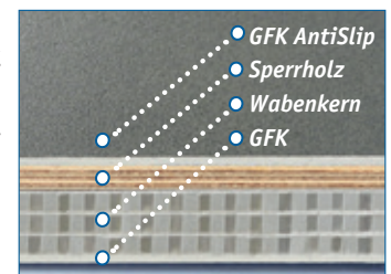
25 mm Boden mit AntiSlip-Oberfläche
